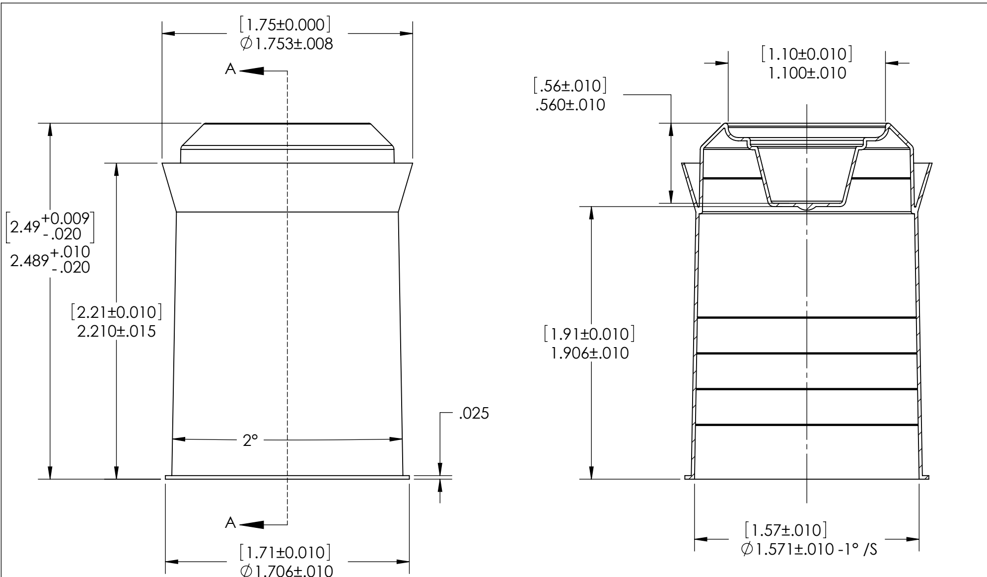
SECTION A-A
